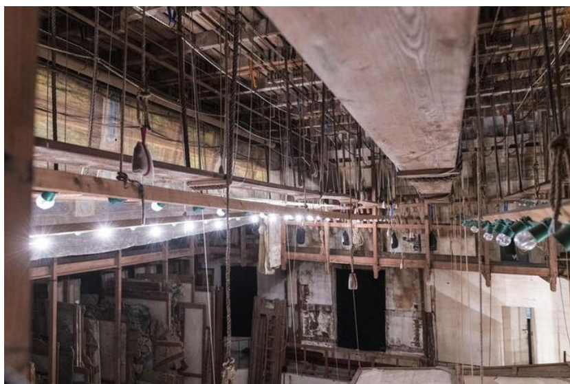
Machinerie de scène © GrandPalaisRmn (Domaine de Compiègne) / Tony Querrec
